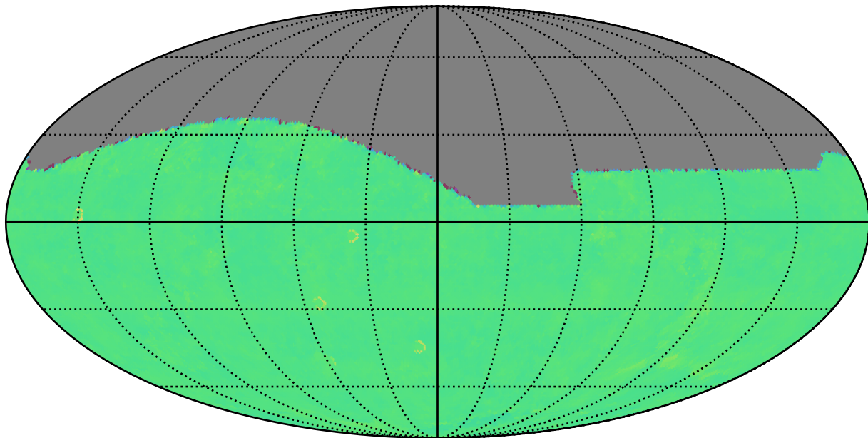
ddf_half_v3.4_10yrs i: Kuiper rotTelPos
