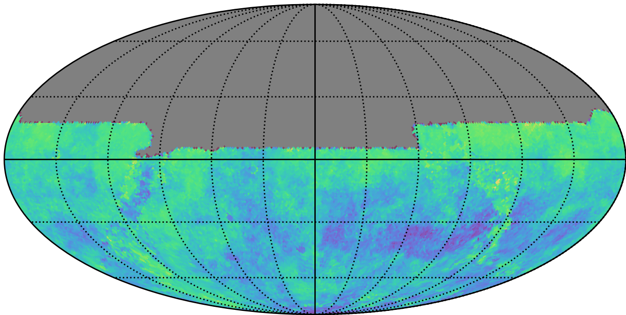
ddf_half_v3.4_10yrs u: Kuiper rotSkyPos
