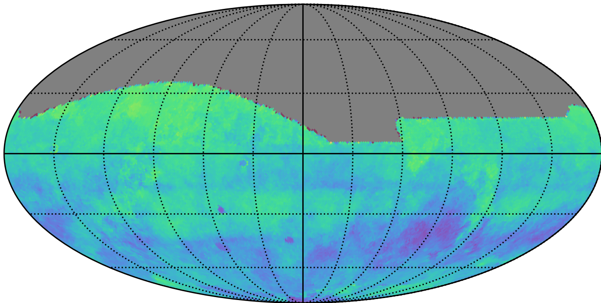
ddf_half_v3.4_10yrs i: Kuiper rotSkyPos
