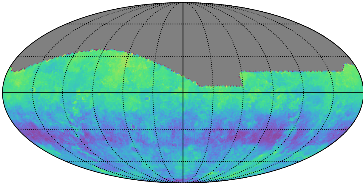
ddf_half_v3.4_10yrs g: Kuiper rotSkyPos
