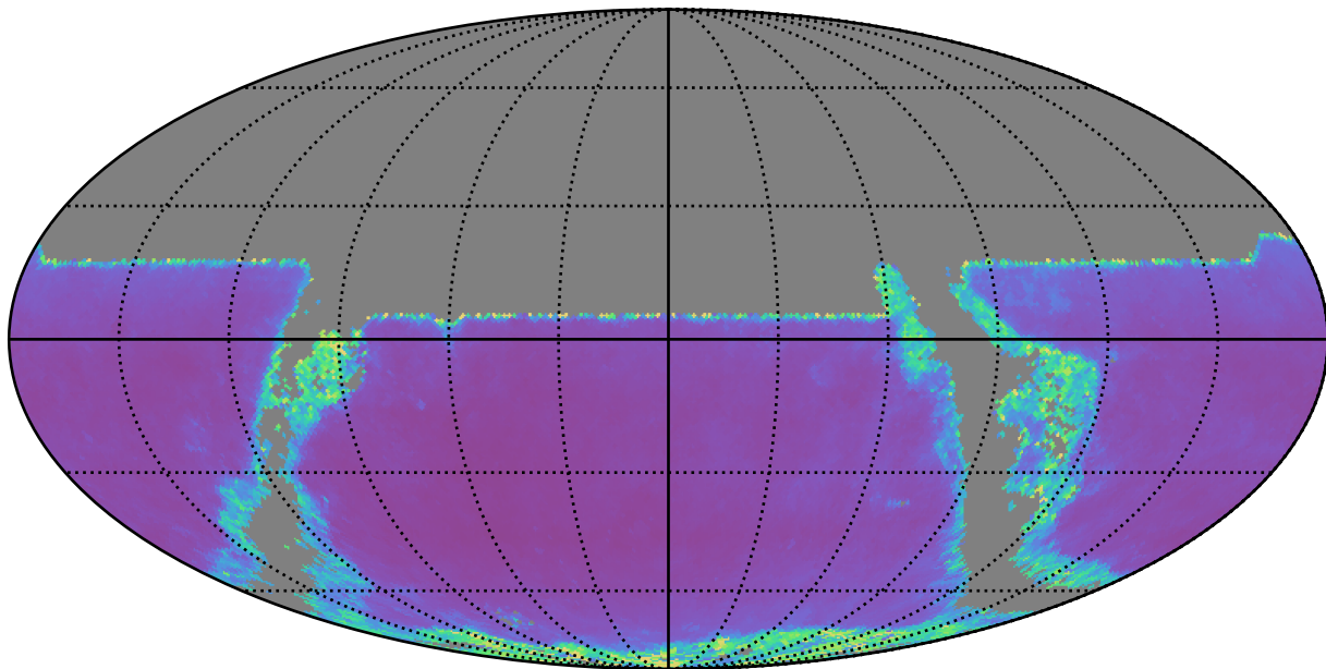
ddf_half_v3.4_10yrs y band: AGN SF_uncert
