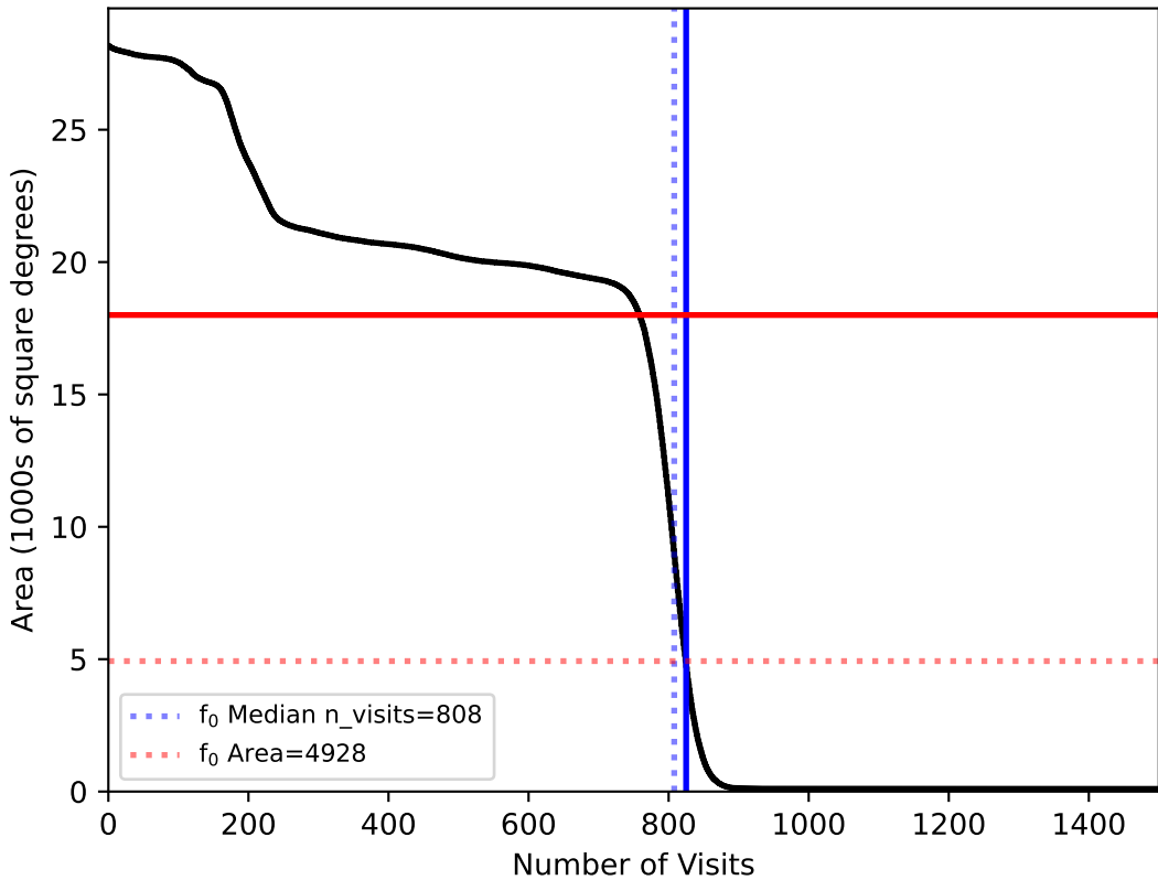
ddf_half_v3.4_10yrs All sky: f0
