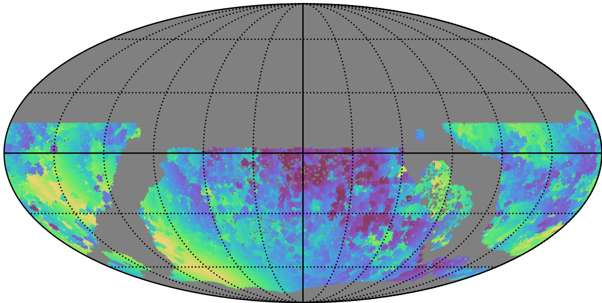
ddf_half_v3.4_10yrs WFD y band: Min solarElong
