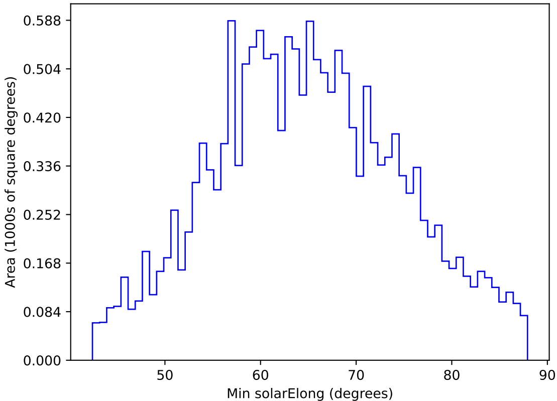
ddf_half_v3.4_10yrs WFD y band: Min solarElong
