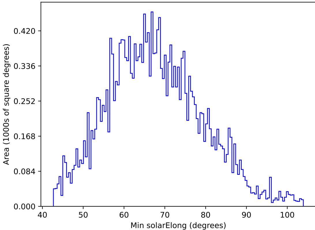
ddf_half_v3.4_10yrs All sky y band: Min solarElong
