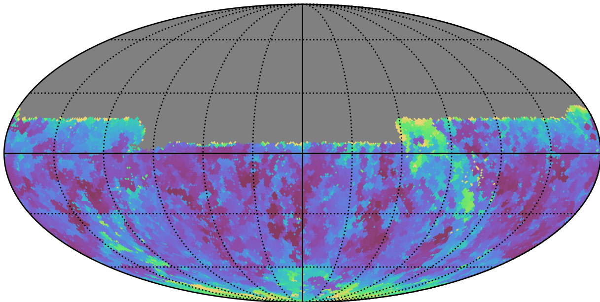
ddf_half_v3.4_10yrs Yr 1 y band: Min seeingGeom
