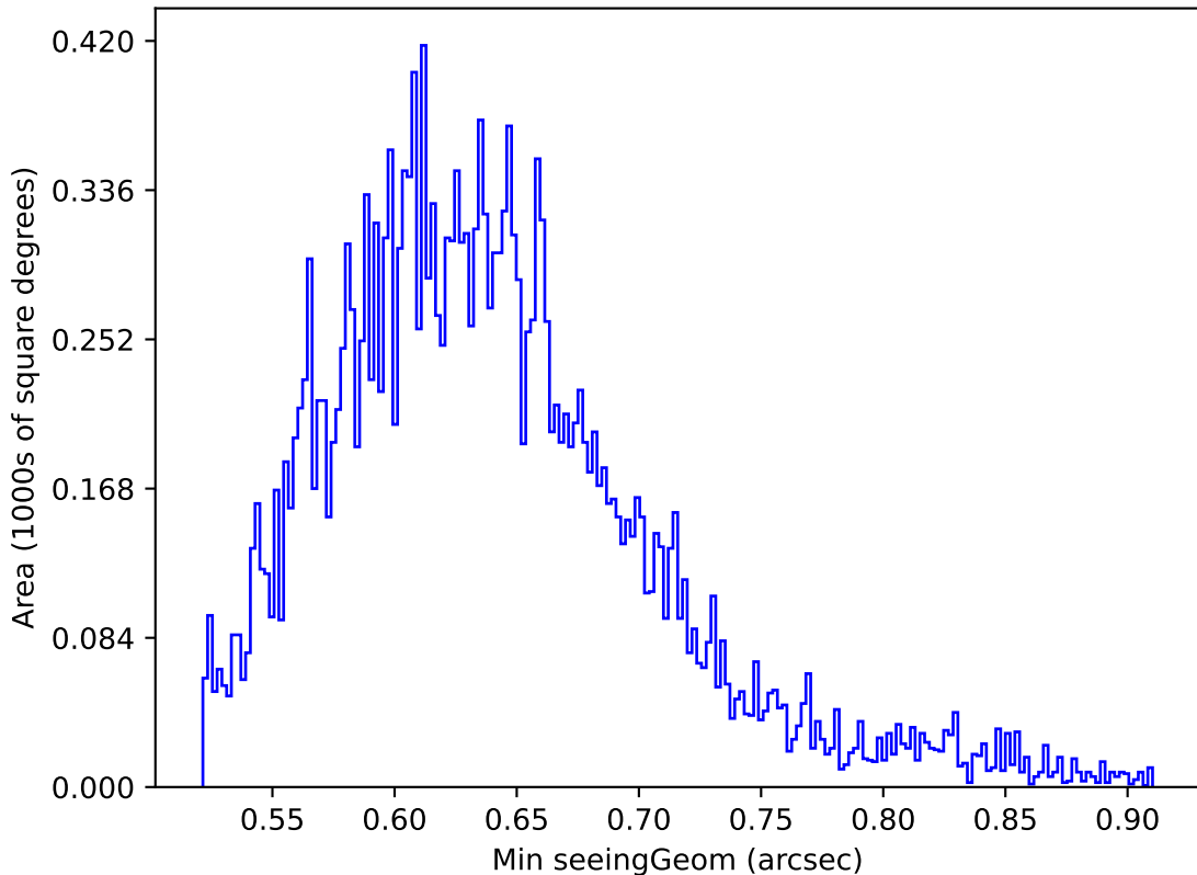
ddf_half_v3.4_10yrs Yr 1 y band: Min seeingGeom
