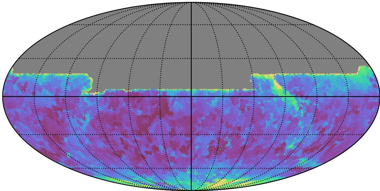
ddf_half_v3.4_10yrs All sky y band: Min seeingEff
