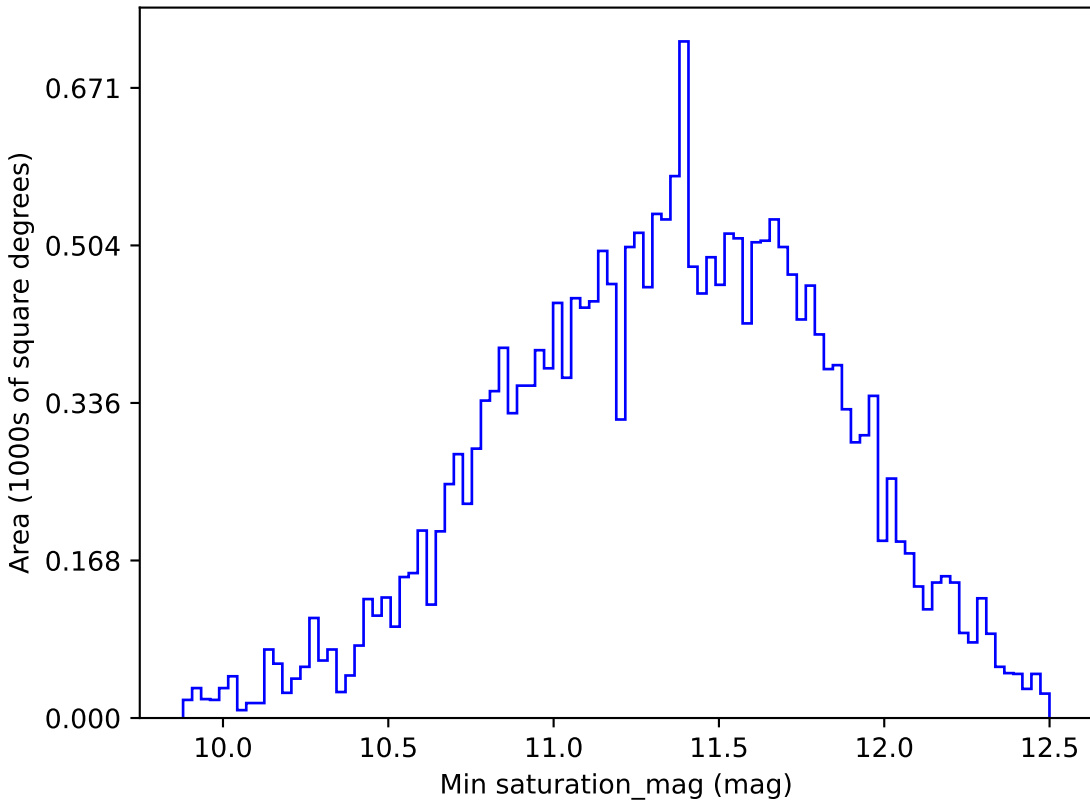
ddf_half_v3.4_10yrs All sky y band: Min saturation_mag
