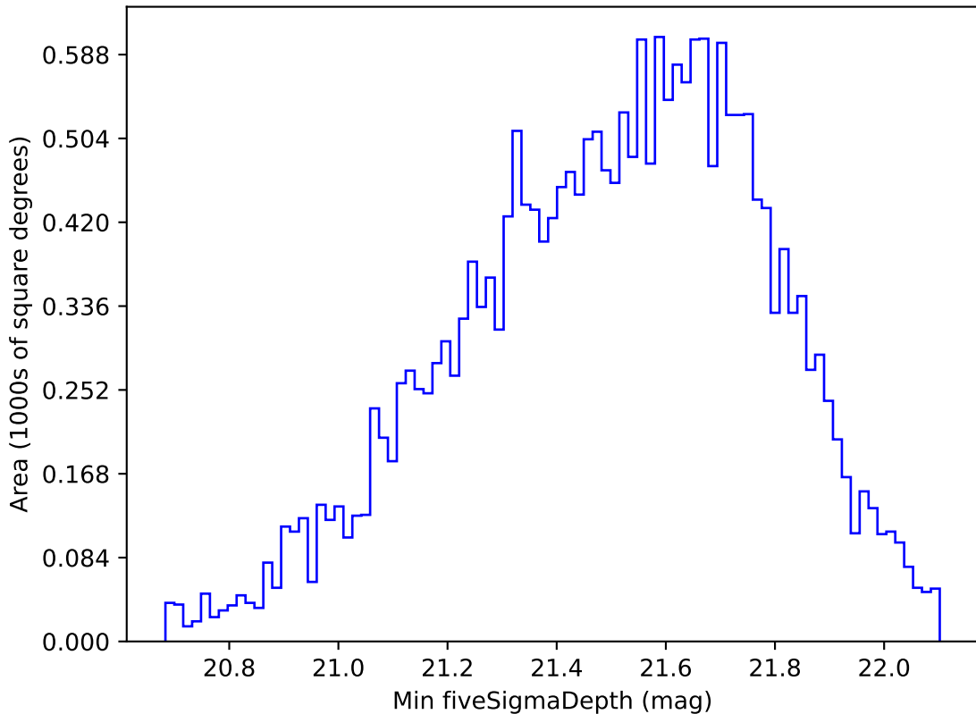
ddf_half_v3.4_10yrs Yr 1 y band: Min fiveSigmaDepth
