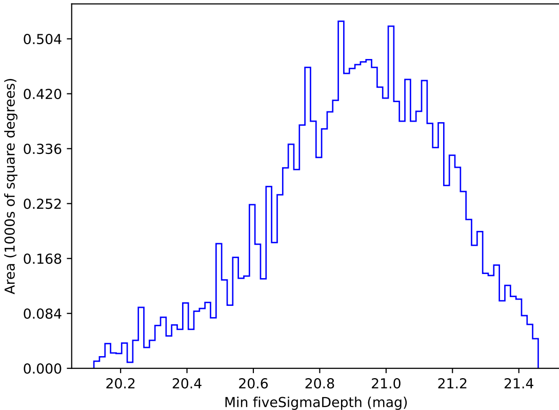
ddf_half_v3.4_10yrs WFD y band: Min fiveSigmaDepth
