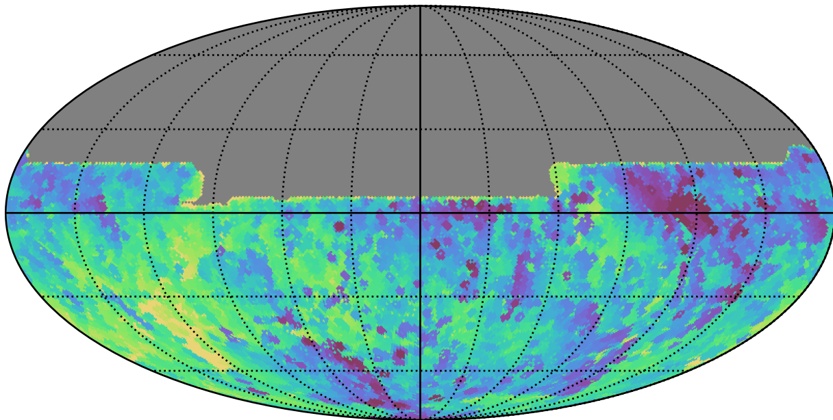
ddf_half_v3.4_10yrs All sky y band: Min fiveSigmaDepth
