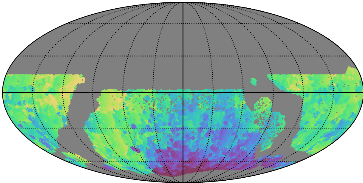
ddf_half_v3.4_10yrs WFD y band: Min HA
