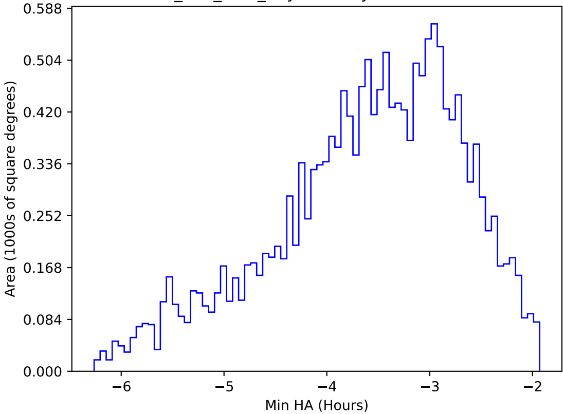
ddf_half_v3.4_10yrs WFD y band: Min HA
