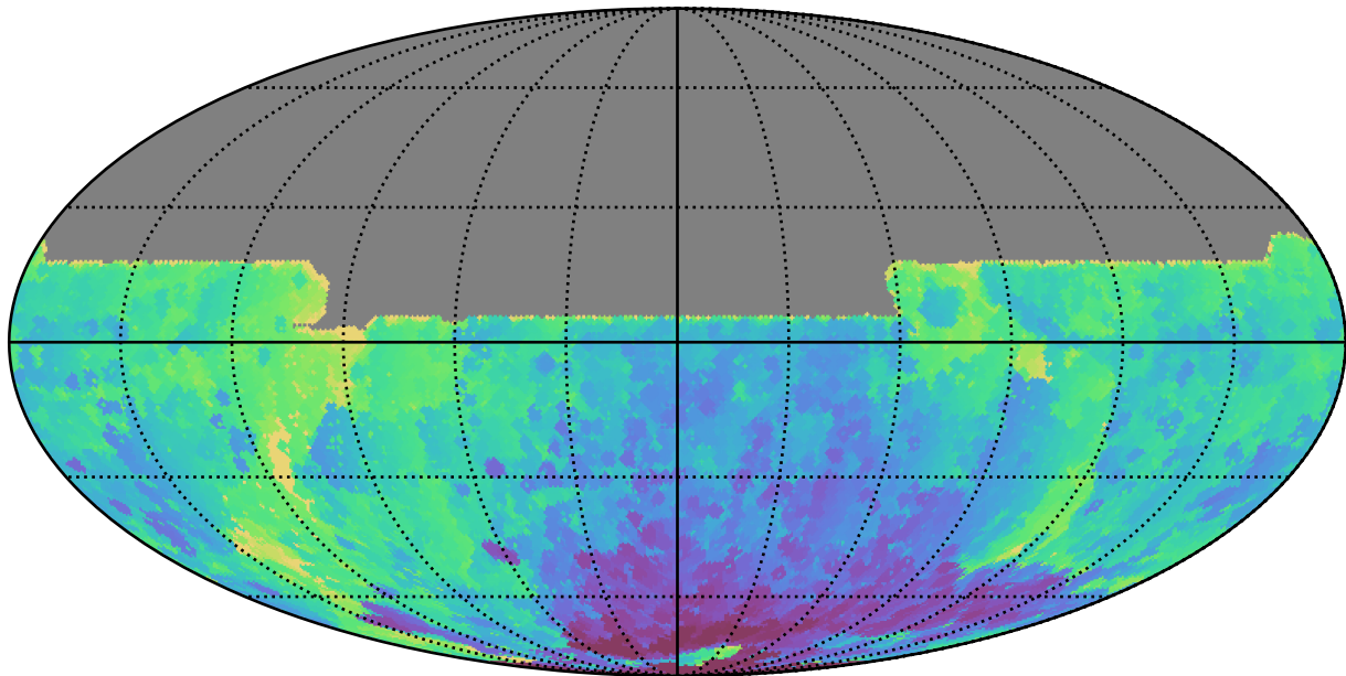
ddf_half_v3.4_10yrs All sky y band: Min HA
