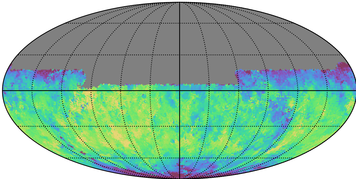
ddf_half_v3.4_10yrs Yr 1 y band: Median fiveSigmaDepth
