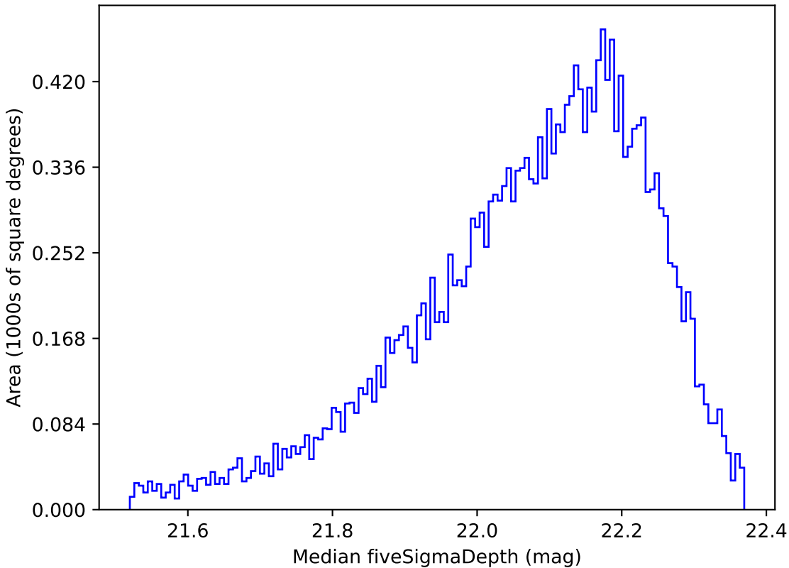
ddf_half_v3.4_10yrs Yr 1 y band: Median fiveSigmaDepth
