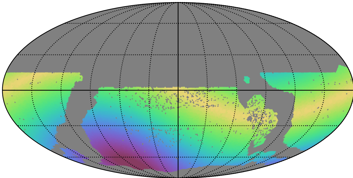
ddf_half_v3.4_10yrs WFD y band: Max solarElong
