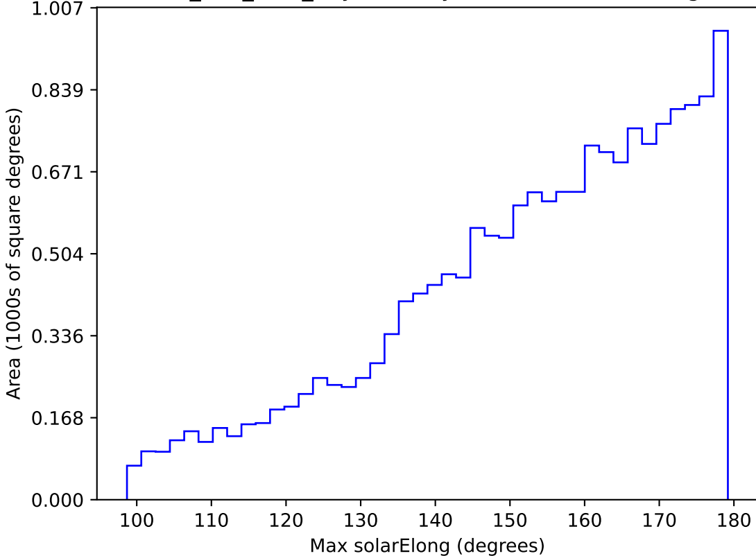
ddf_half_v3.4_10yrs WFD y band: Max solarElong
