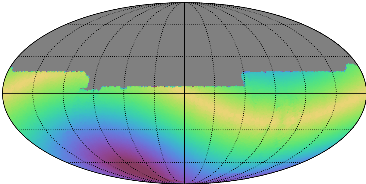
ddf_half_v3.4_10yrs All sky y band: Max solarElong
