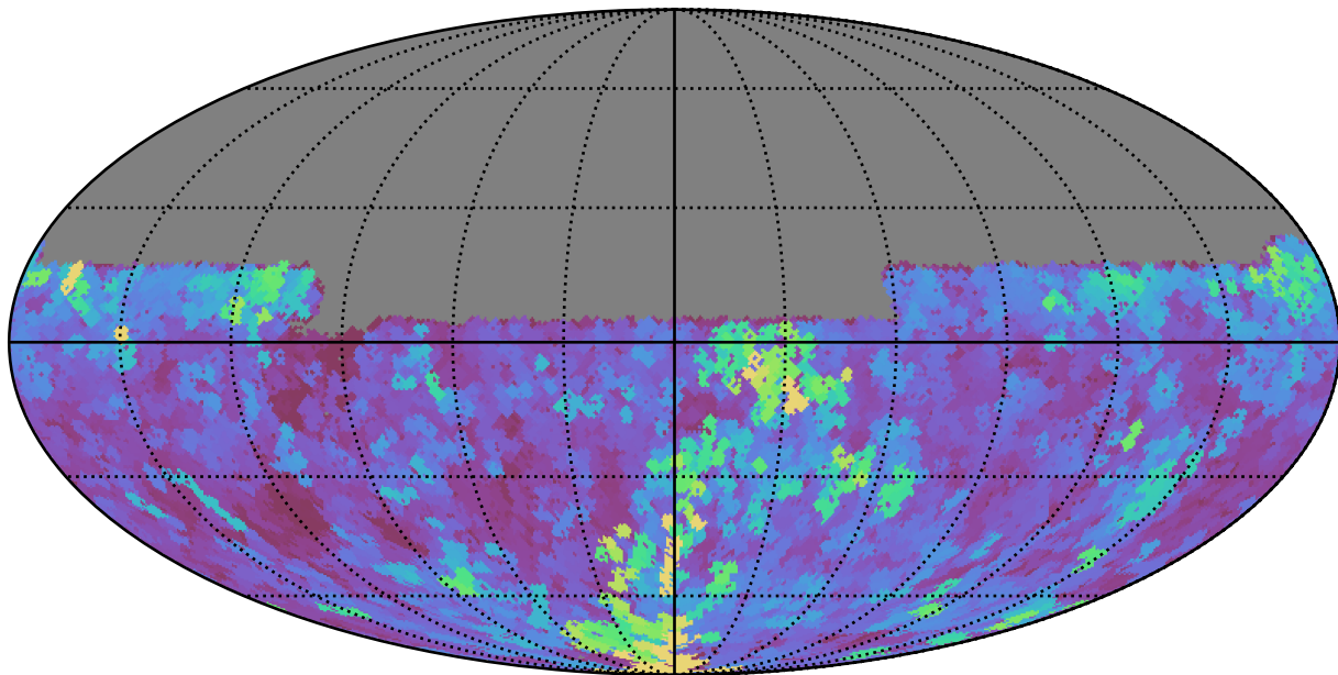
ddf_half_v3.4_10yrs Yr 1 y band: Max seeingGeom
