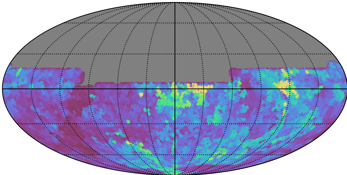
ddf_half_v3.4_10yrs All sky y band: Max seeingEff
