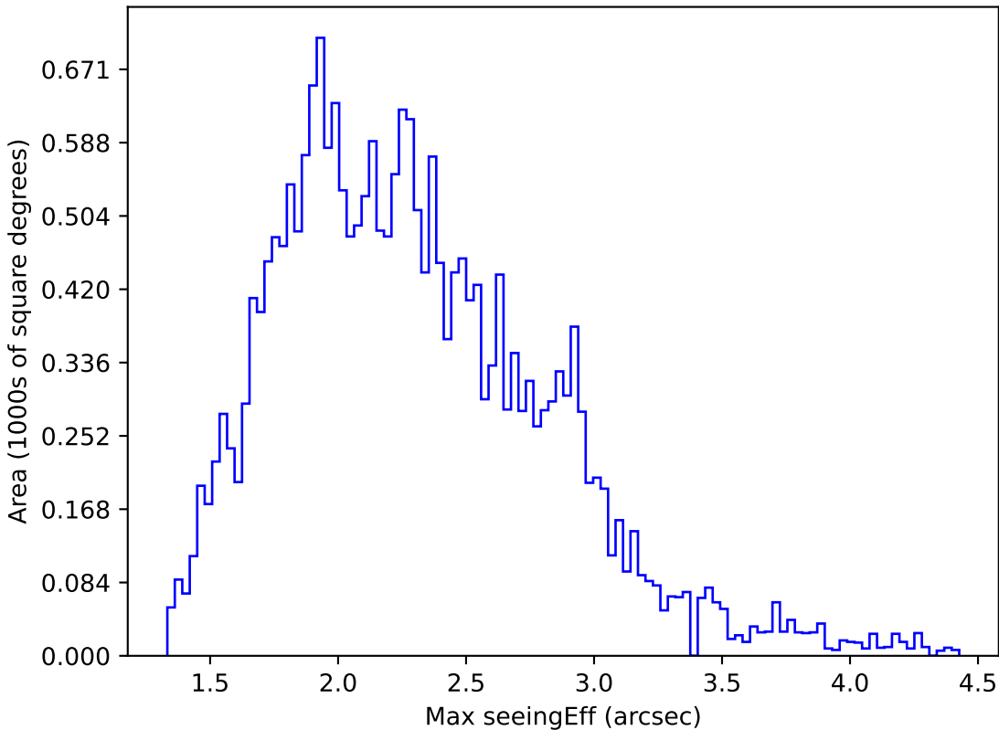
ddf_half_v3.4_10yrs All sky y band: Max seeingEff
