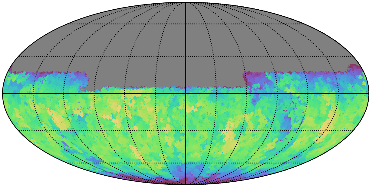
ddf_half_v3.4_10yrs Yr 1 y band: Max fiveSigmaDepth
