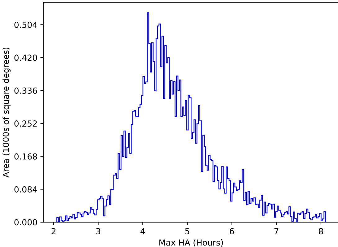
ddf_half_v3.4_10yrs All sky y band: Max HA
