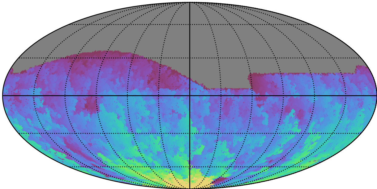
ddf_half_v3.4_10yrs All sky g band: Max HA
