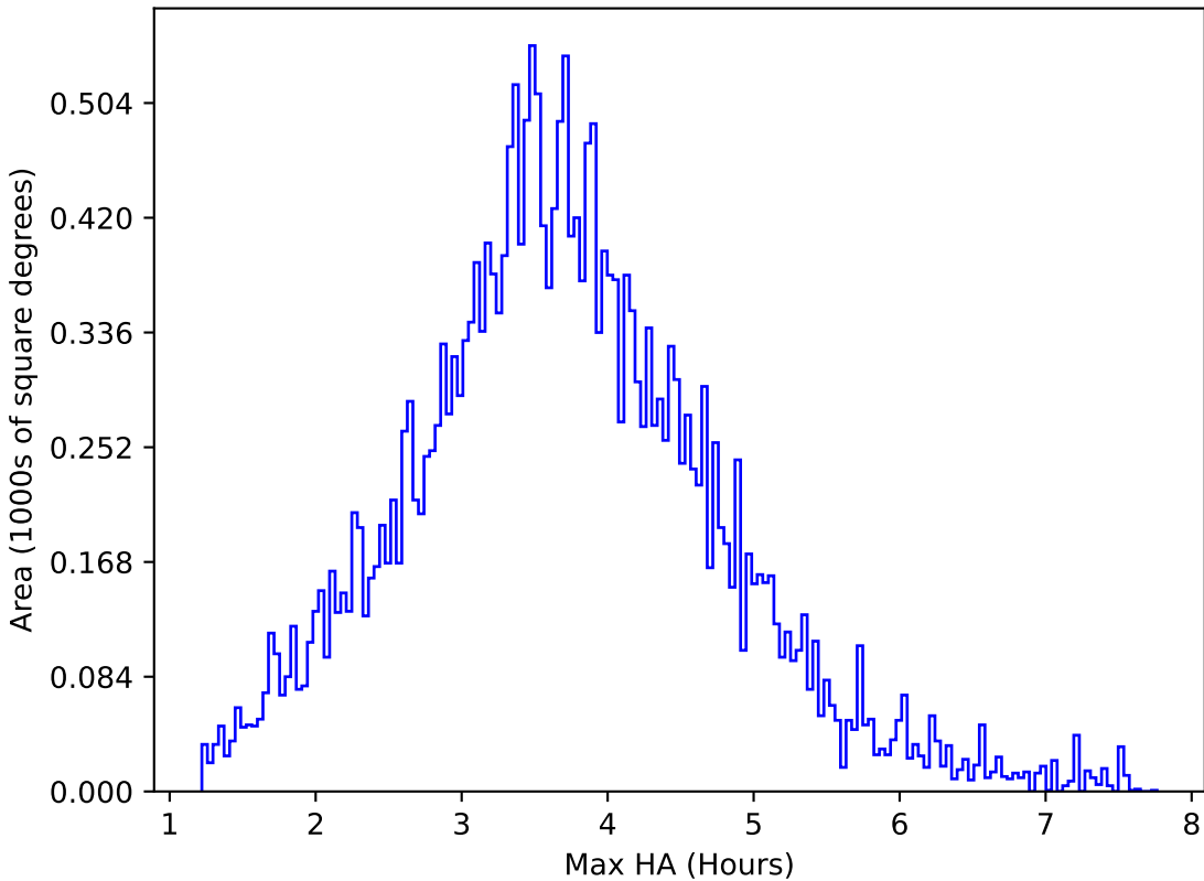
ddf_half_v3.4_10yrs All sky g band: Max HA
