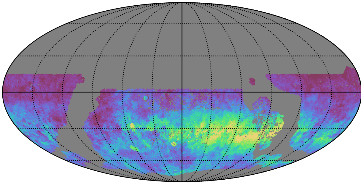
ddf_half_v3.4_10yrs WFD y band: AngleRms rotSkyPos
