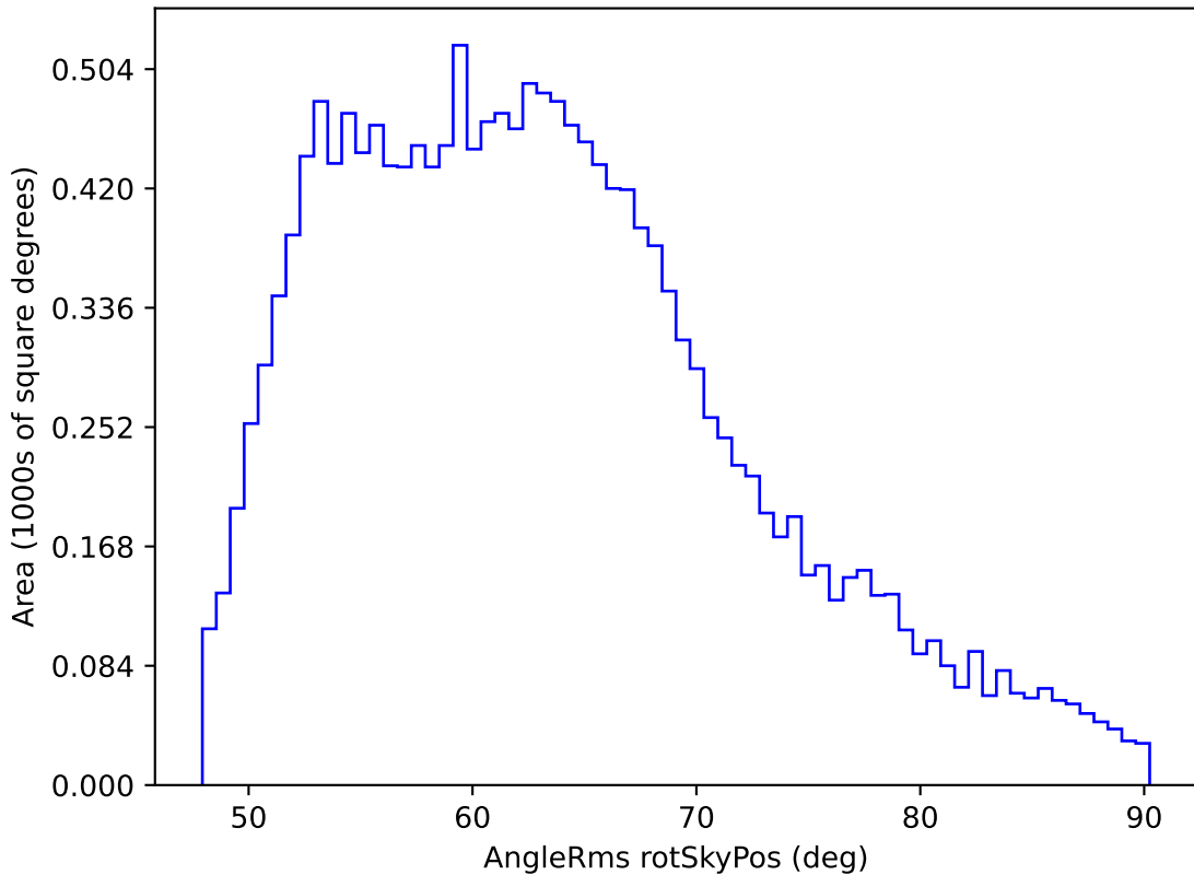
ddf_half_v3.4_10yrs WFD y band: AngleRms rotSkyPos
