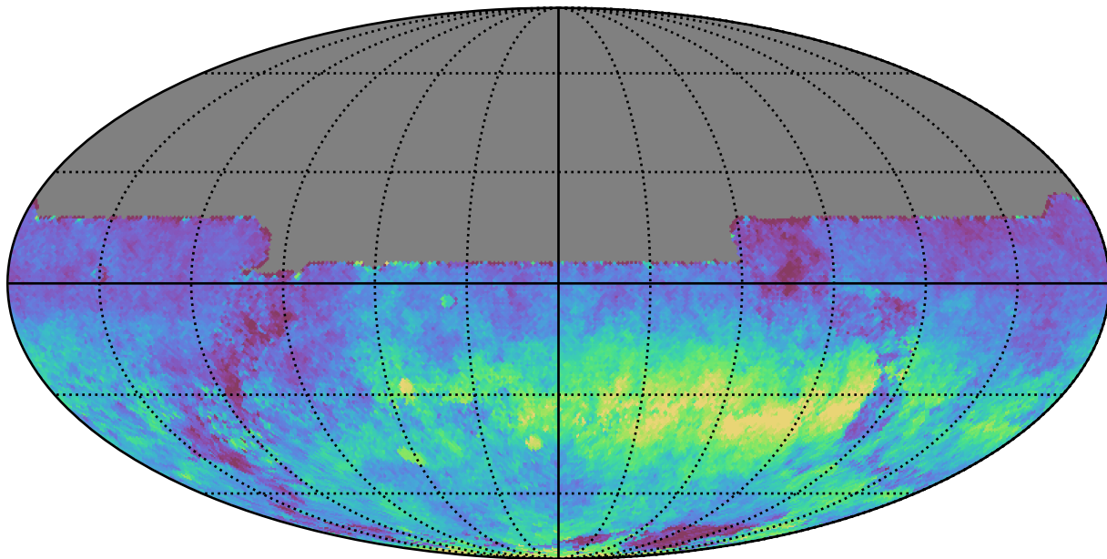
ddf_half_v3.4_10yrs All sky y band: AngleRms rotSkyPos
