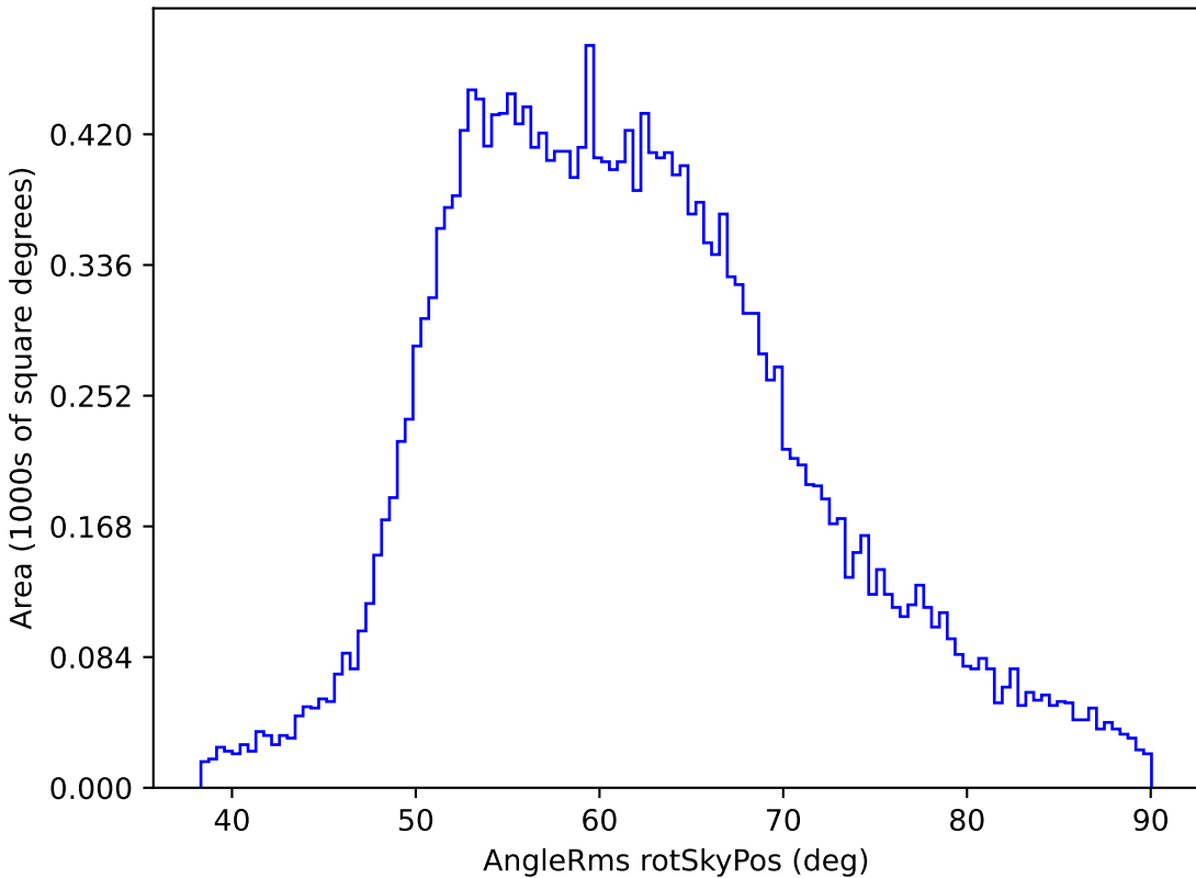
ddf_half_v3.4_10yrs All sky y band: AngleRms rotSkyPos
