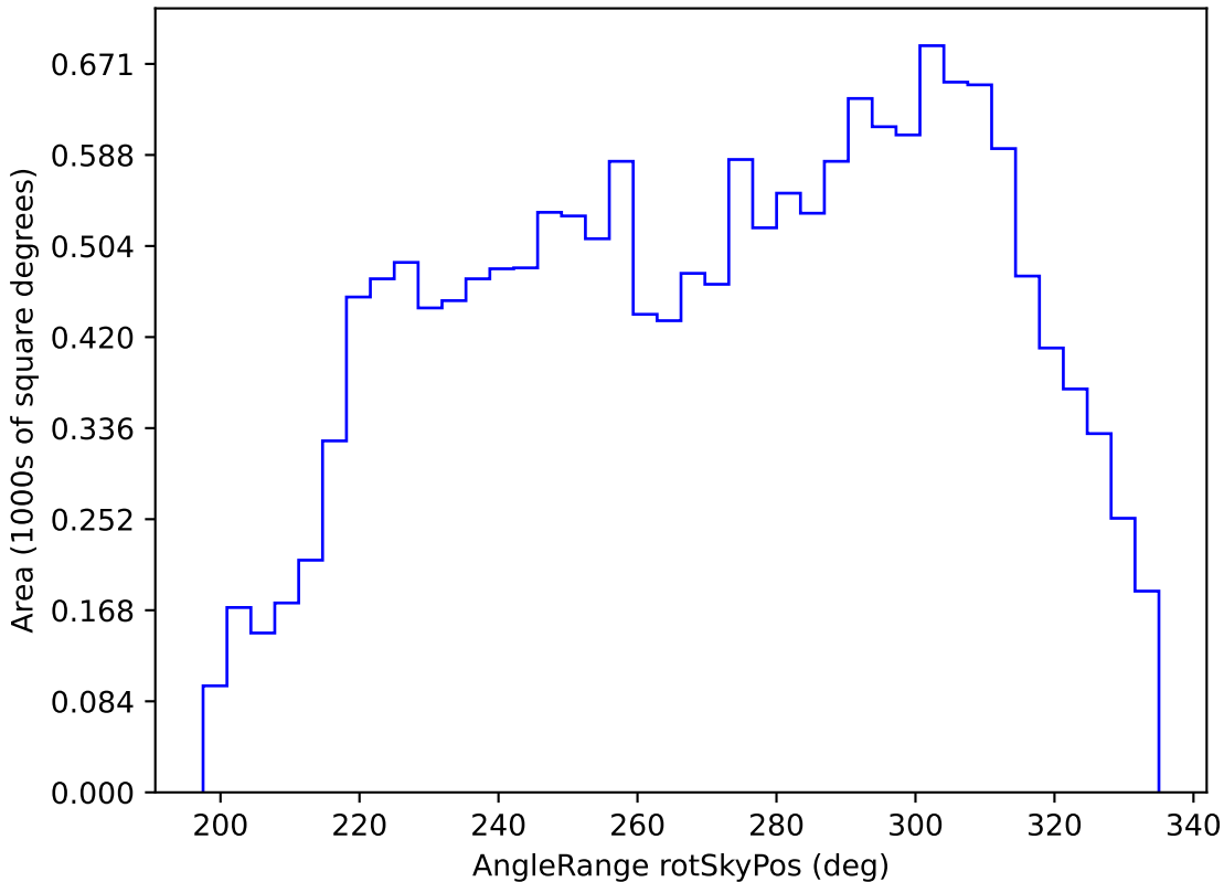
ddf_half_v3.4_10yrs WFD y band: AngleRange rotSkyPos
