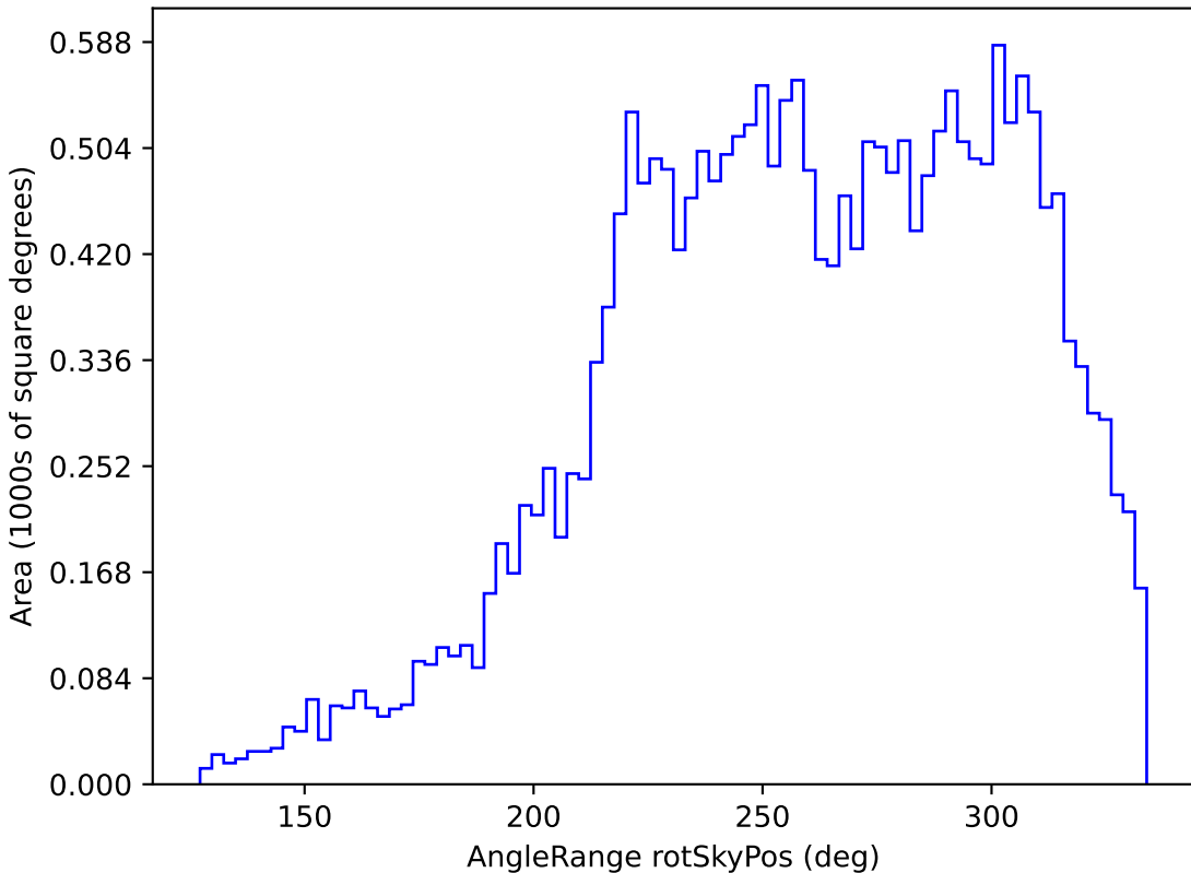
ddf_half_v3.4_10yrs All sky y band: AngleRange rotSkyPos
