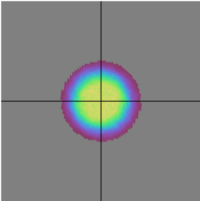
ddf_half_v3.4_10yrs u band: DD:ELAISS1 NVisits
