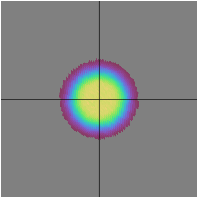
ddf_half_v3.4_10yrs r band: DD:ELAISS1 NVisits
