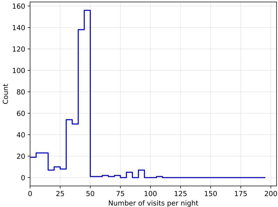
ddf_half_v3.4_10yrs all bands: DD:ELAISS1 NVisitsPerNight
