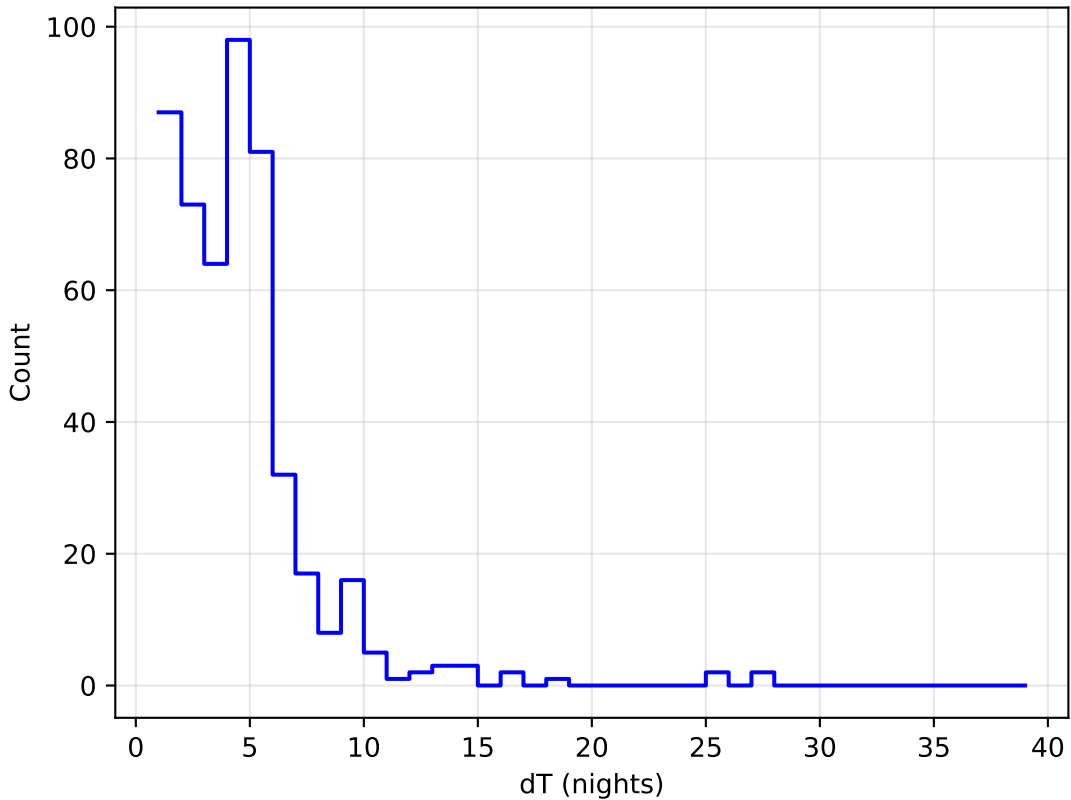
ddf_half_v3.4_10yrs all bands: DD:ELAISS1 Delta Nights Histogram
