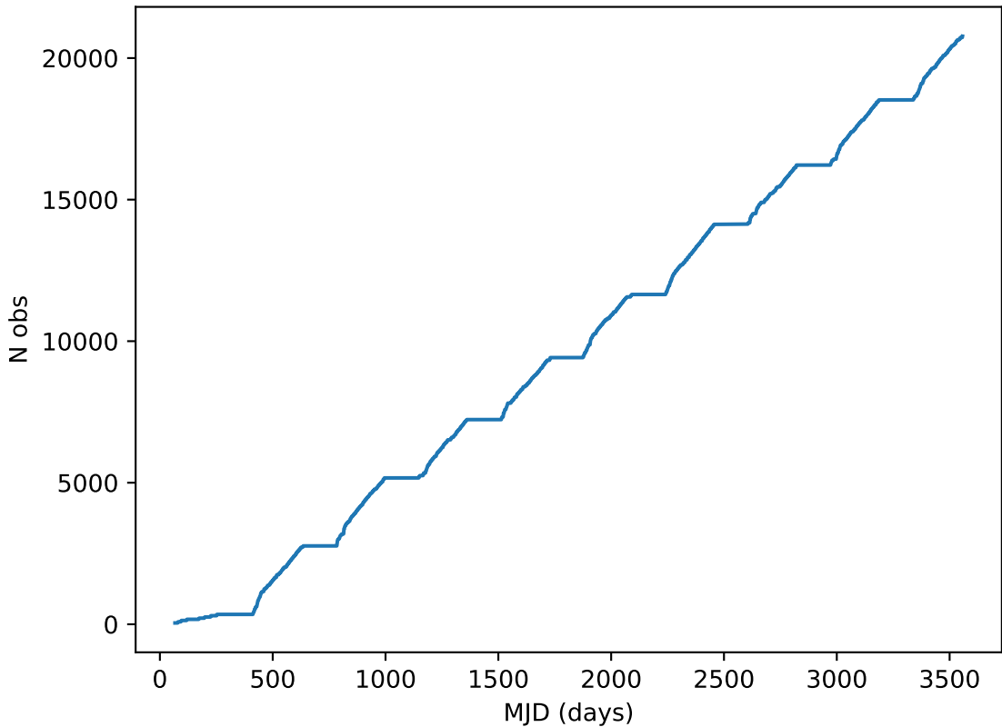
ddf_half_v3.4_10yrs all bands: DD:ELAISS1 Cumulative NVisits
