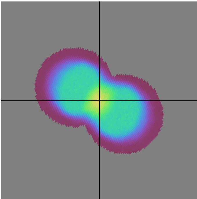
ddf_half_v3.4_10yrs y band: DD:EDFS NVisits
