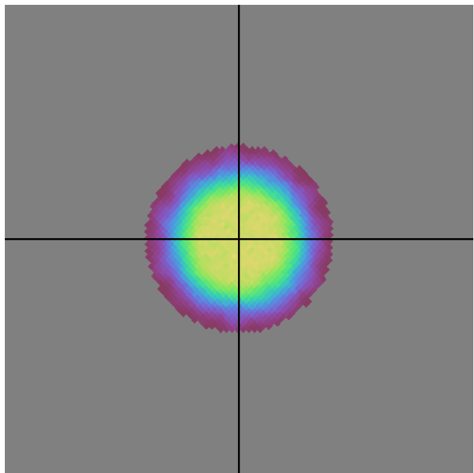
ddf_half_v3.4_10yrs y band: DD:ECDFS NVisits
