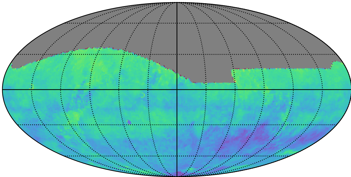
ddf_acor_sf30_lsf40_lsr50_v3.4_10yrs i: Kuiper rotSkyPos
