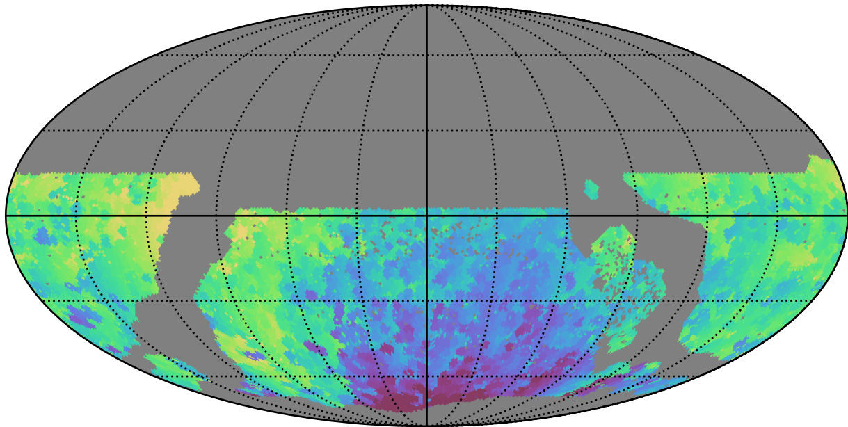
ddf_acor_sf30_lsf40_lsr50_v3.4_10yrs WFD y band: Min HA
