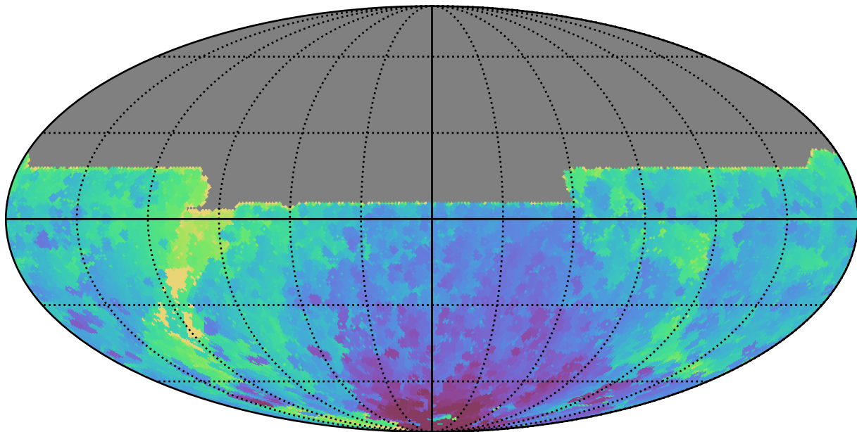
ddf_acor_sf30_lsf40_lsr50_v3.4_10yrs All sky y band: Min HA
