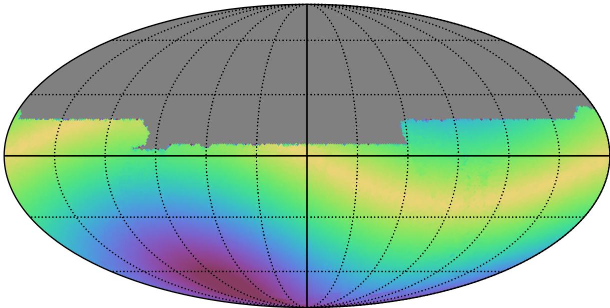
ddf_acor_sf30_lsf40_lsr50_v3.4_10yrs All sky y band: Max solarElong
