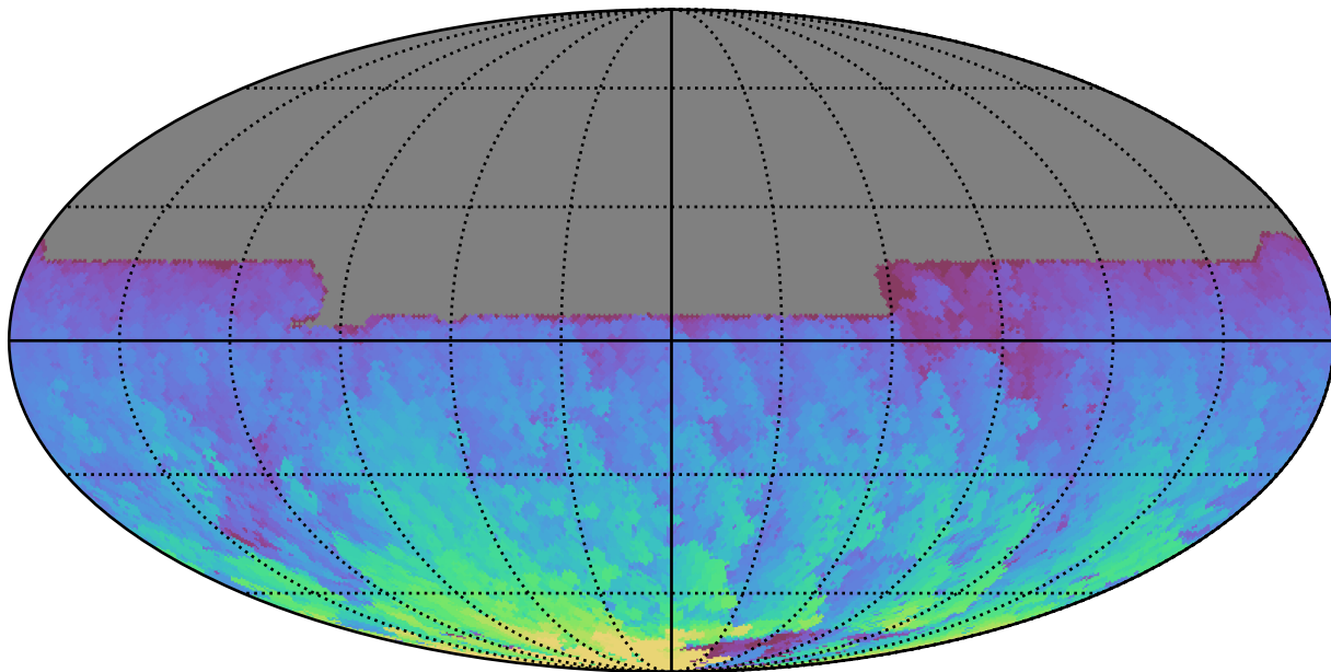
ddf_acor_sf30_lsf40_lsr50_v3.4_10yrs All sky y band: Max HA
