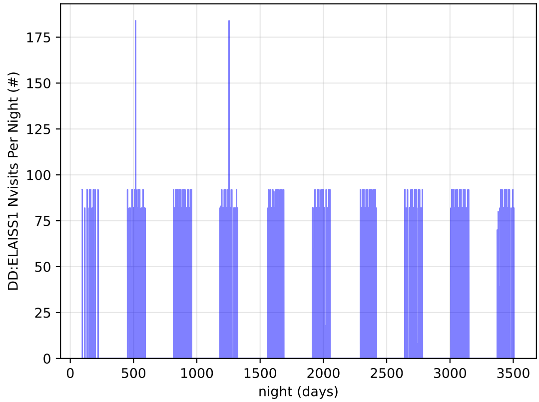
ddf_acor_sf30_lsf40_lsr50_v3.4_10yrs all bands: DD:ELAISS1 Nvisits Per Night
